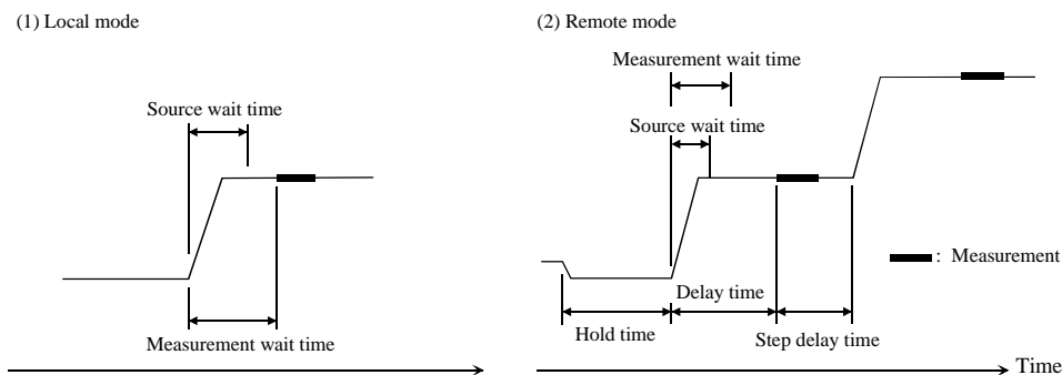
Figure 6-9 出力／測定ウェイト時間
