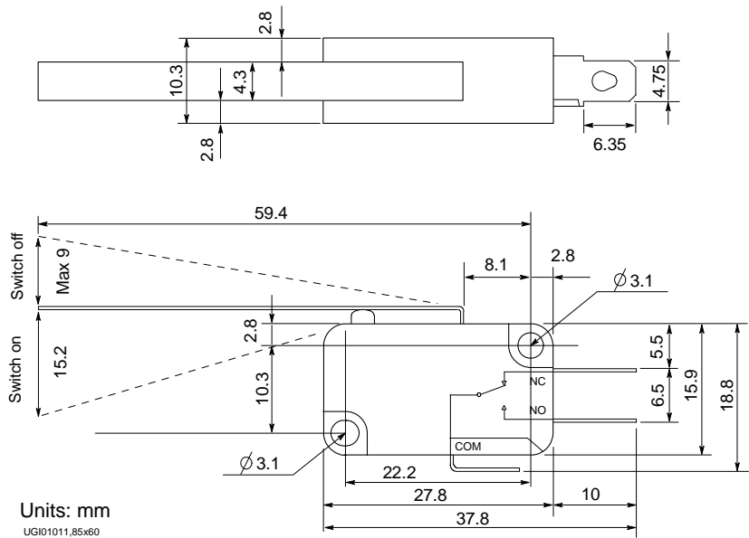
Figure 3-9 インターロック・スイッチの寸法 (Agilent 部品番号 3101-0302)
