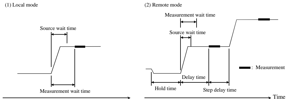
Figure 4-1 出力／測定ウエイト時間
