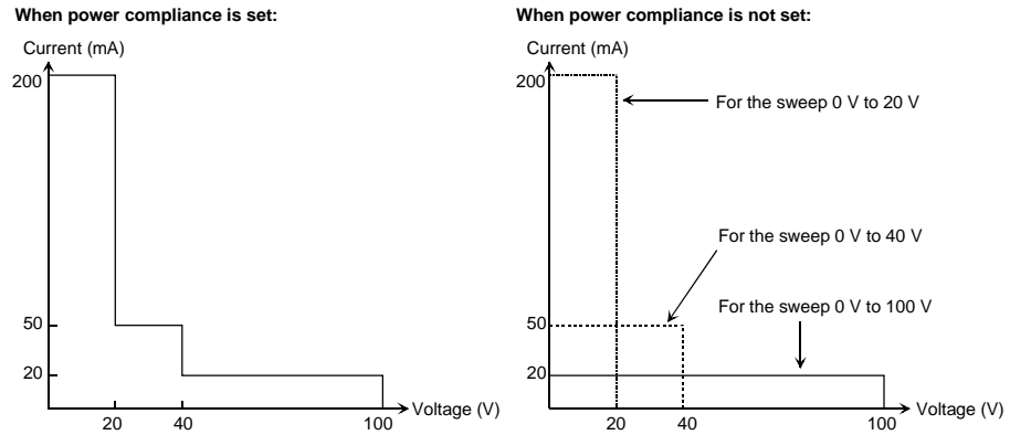
Figure 6-5 MPSMU で電圧掃引を行う場合の電流範囲
