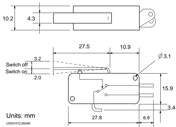
Figure 3-10 インターロック・スイッチの寸法 (Agilent 部品番号 3101-3241)
