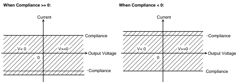
Figure 6-2 コンプライアンスと出力の関係 (DV、マニュアル極性モード)
