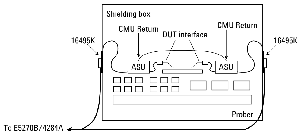
ASU の設置イメージ
