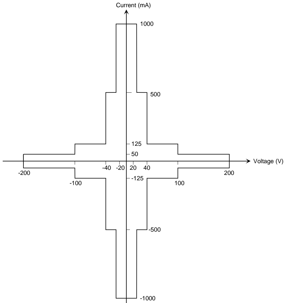
HPSMU 出力／測定範囲
