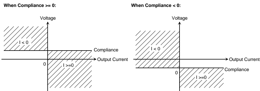
Figure 6-3 コンプライアンスと出力の関係 (DI、マニュアル極性モード)
