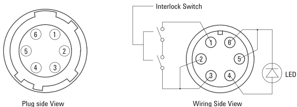
Figure 3-7 インターロック・コネクタのピン配置
